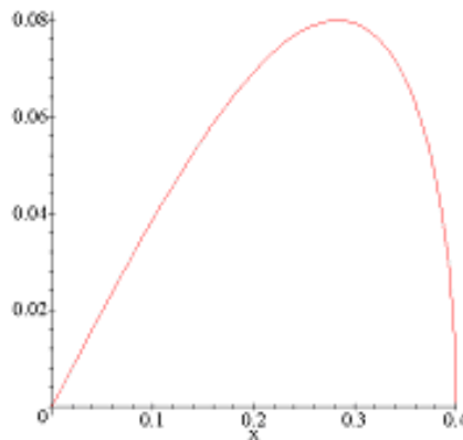
7.12. ábra. A T függvény grafikonja a 11. feladatban
