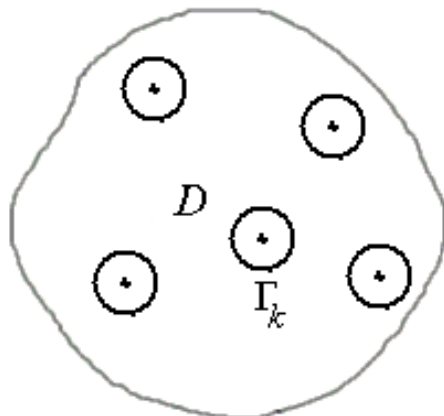
10.6. ábra. Vázlat a reziduúmtétel bizonyításához
