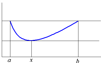
7.2. ábra. A Rolle-tétel szemléltetése
