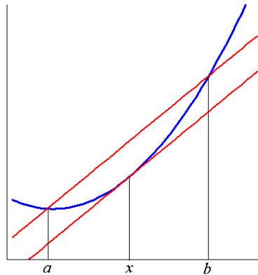
7.3. ábra. A Lagrange-középértéktétel szemléltetése
