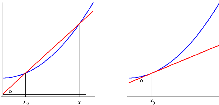
7.1. ábra. \operatorname{tg} \alpha = \frac{f(x) - f(x_0)}{x - x_0}
