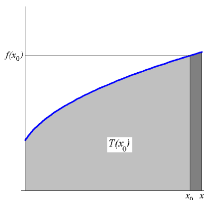
9.1. ábra. A T területfüggvény és megváltozása
