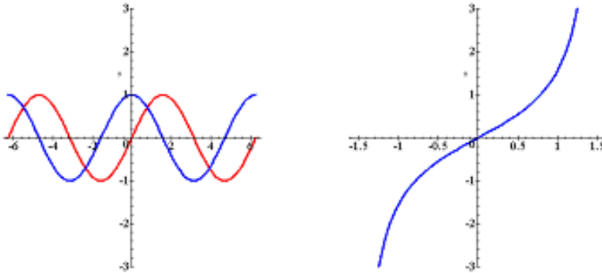
6.4. ábra. Az x \mapsto \sin x , x \mapsto \cos x és az x \mapsto \operatorname{tg} x függvény grafikonja
