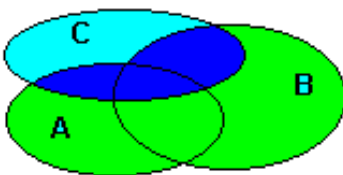
2.4. ábra. Az 1. disztributivitás szemléltetése Venn-diagrammokkal.
