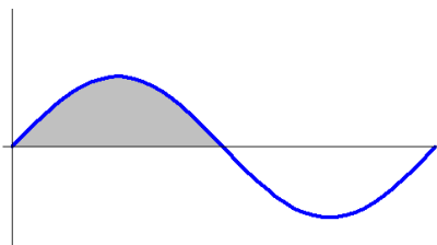
9.5. ábra. Fél szinuszhullám alatti terület
